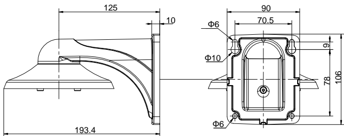
墙装支架
