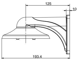
图2-14-1 尺寸图
