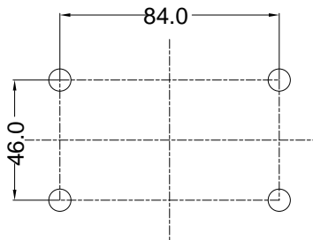
图 2-7-2 摄像机安装孔位示意图
