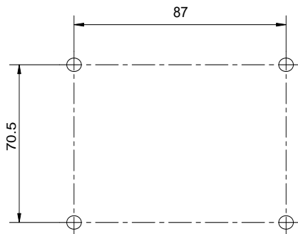
图 2-14-2 摄像机安装孔位示意图
