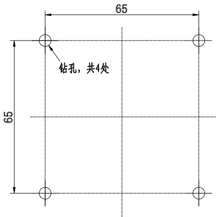
图 2-10-1 安装孔位示意图
