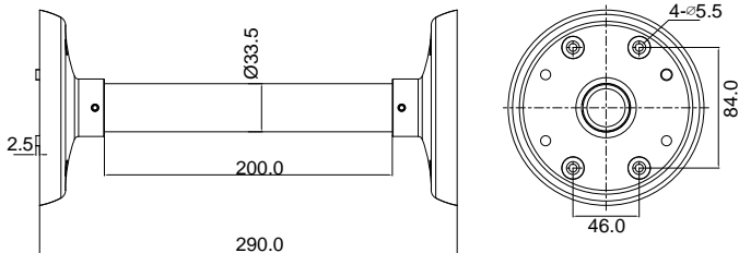
吊装支架
