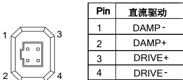
图 2-9-2 引脚标志
