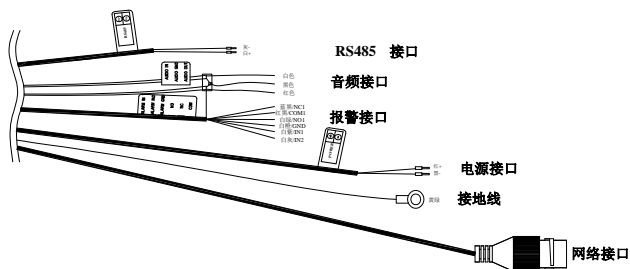
图2-1 标准线缆
