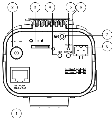
图 2-9-1 接口示意图
