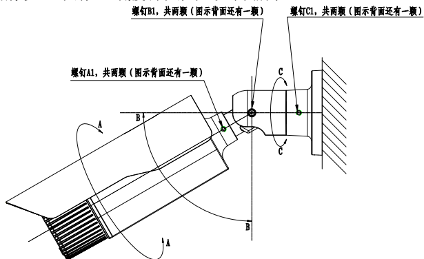
图 2-10-3 墙面装摄像机角度调节
