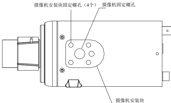
图 2-9-3 摄像机安装块示意图
