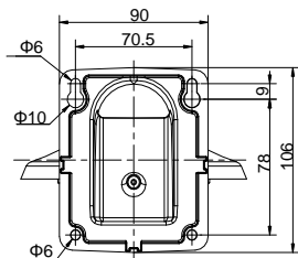
墙装支架
