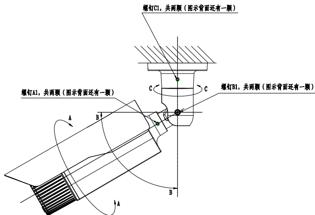
图 2-10-4 吊装摄像机角度调节
