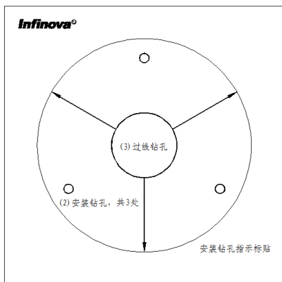
图 2-12-1 安装标贴的示意
