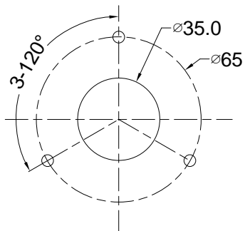
图 2-13-1 摄像机安装孔位示意图
